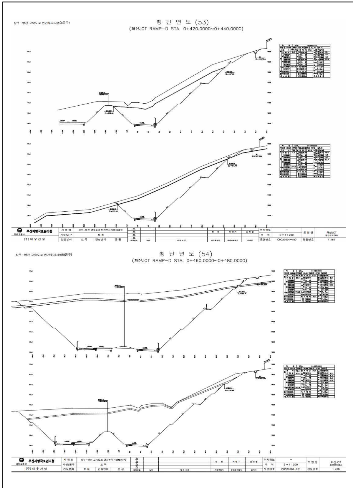
【그림 61.4】 표준횡단면도
