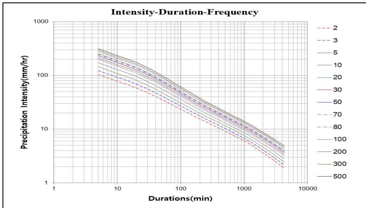
【그림 61.9】 영천지역 IDF곡선
