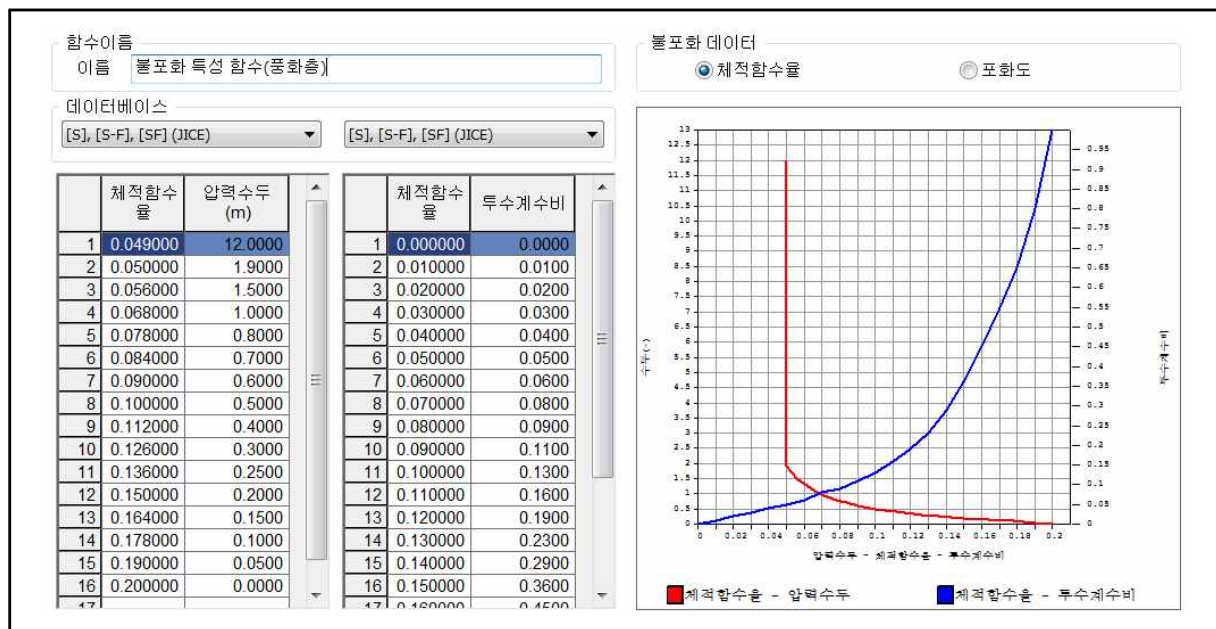
【그림 61.15】 압력수두-체적함수율(포화도)-투수계수비 함수
